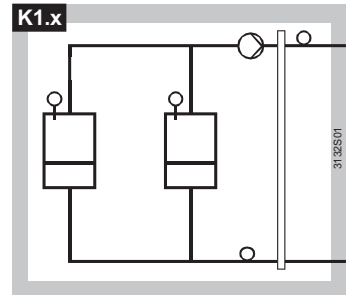
Многокотельная установка: - 1 основной насос на подаче
