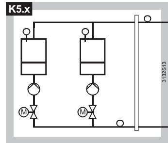
Многокотельная установка: - 1 насос на обратке котлов - 1 отсеchnый клапан на обратке котлов
