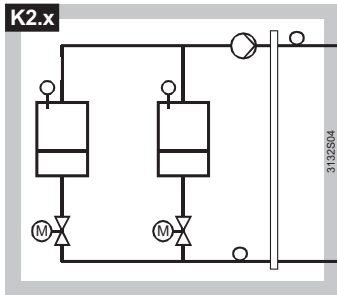
Многокотельная установка: - 1 основной насос на подаче - 1 отсеchnый клапан на обратке котлов
