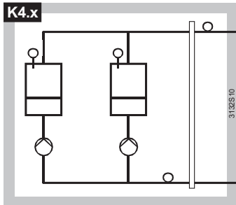
Многокотельная установка: - 1 насос на обратке котлов
