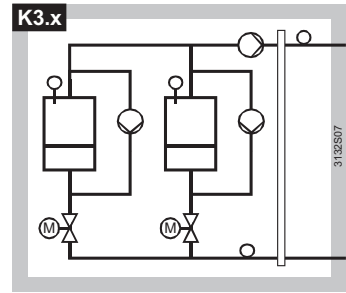
Многокотельная установка: - 1 основной насос на подаче - 1 насос на байпасе котлов - 1 отсеchnый клапан на обратке котлов
