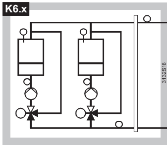
Многокотельная установка: - 1 насос на обратке котлов - Поддержание теплоносителя в обратном трубопроводе котлов при помощи смеси-тельных клапанов
