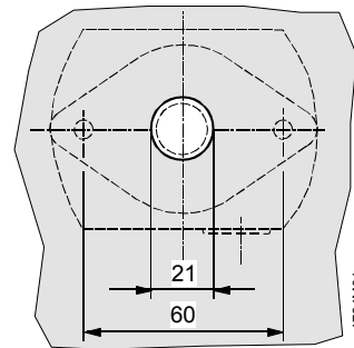
Шаблон для сверления
