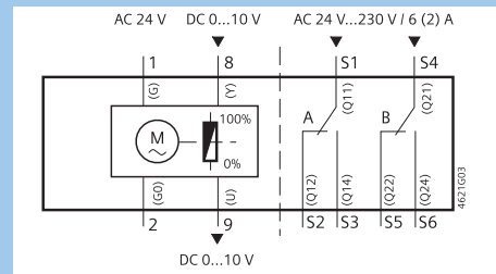
Модулирующий (0...10 В пост. тока), 24 В пер. тока
