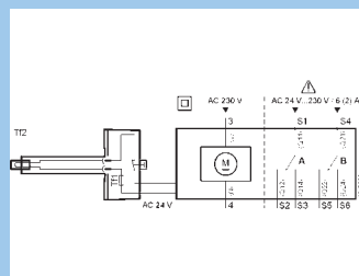
2-позиционный, 230 В пер. тока
