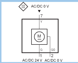
Вкл/Выкл (1-проводной однополюсный на одно направление), 24 В пер./пост. тока
